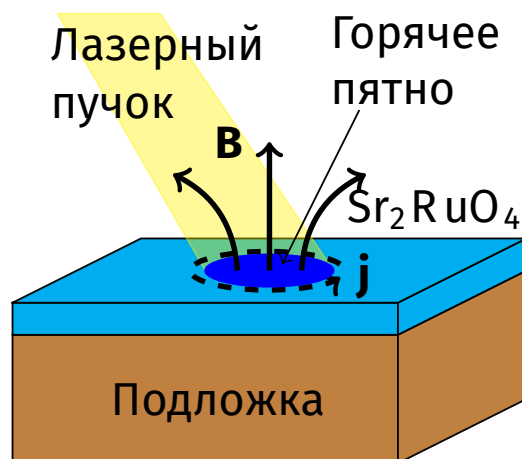
Рис. 1: Предлагаемая схема эксперимента. Лазерный пучок нагревает образец, создавая сверхпроводящий ток вокруг области с подавленной сверхпроводимостью. Магнитное поле \mathbf{B} , создаваемое током \mathbf{j} , может быть измерено с помощью датчиков Холла или СКВИД микроскопов.
