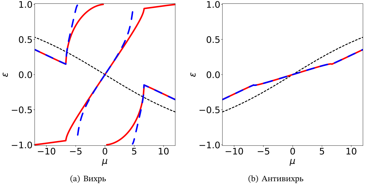
Рис. 2: Квазичастичный спектр для вихрей противоположной ориентации. Здесь \mu — орбитальный момент квазичастицы, \varepsilon \cdot \Delta_0 — ее энергия, где \Delta_0 — величина сверхпроводящей щели вдали от вихря. Численное решение обозначено красными сплошными линиями, синие пунктирные линии соответствуют результату пертурбативного подхода. Черная пунктирная линия соответствует спектральной ветви Кароли-де Жена – Матрикона для свободного вихря [56]. Радиус дефекта R = 0.4\xi , (k_F\xi)^{-1} = 0.06 , \xi — длина когерентности, \hbar k_F — импульс Ферми.
