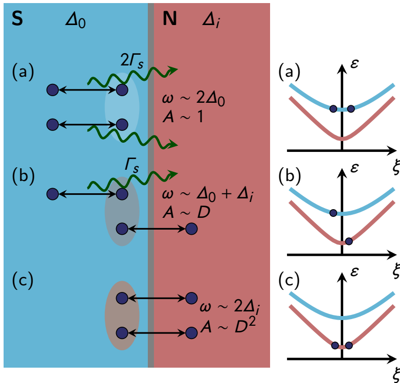
Рис. 3: Схематическая иллюстрация трех сценариев расщепления куперовских пар в SIN систем, которые дают моды Хиггса с различными частотами, скоростями затухания и амплитудами.
